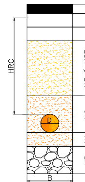
ZANJA DE INSTALACIÓN CON MEJORAMIENTO DE SUELO EN PIEDRA RAJÓN
