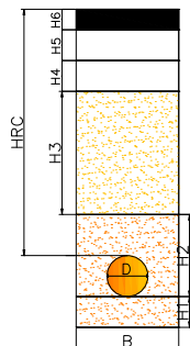
VIA VEHICULAR PAVIMENTO FLEXIBLE Y RÍGIDO
